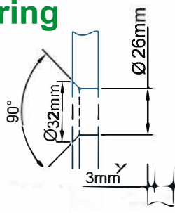
Forsænket hul
