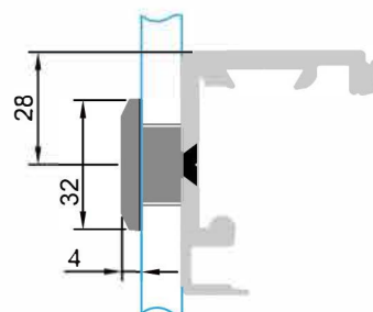
Fladt hul
