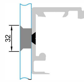
Forsænket hul
